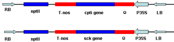
图 3 CpTI 转化载体
